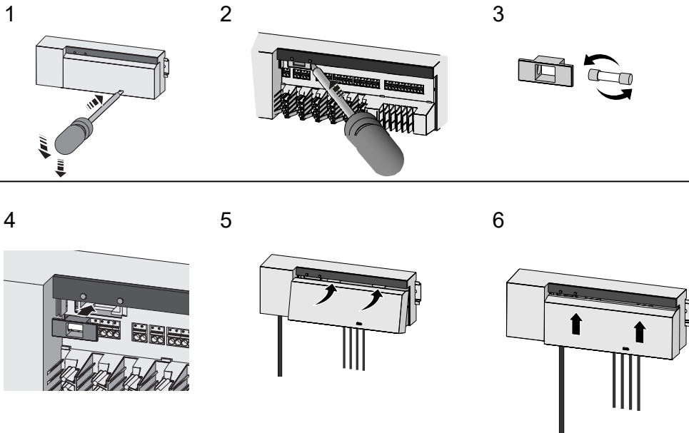
Afb. 7: Zekering van het Basisstation vervangen
